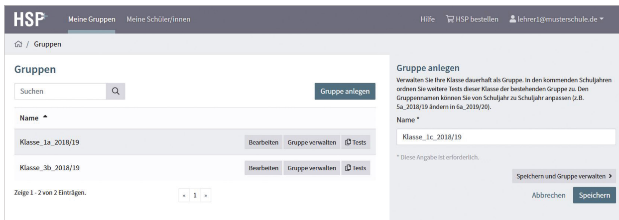
Abb. 3 Gruppe anlegen
